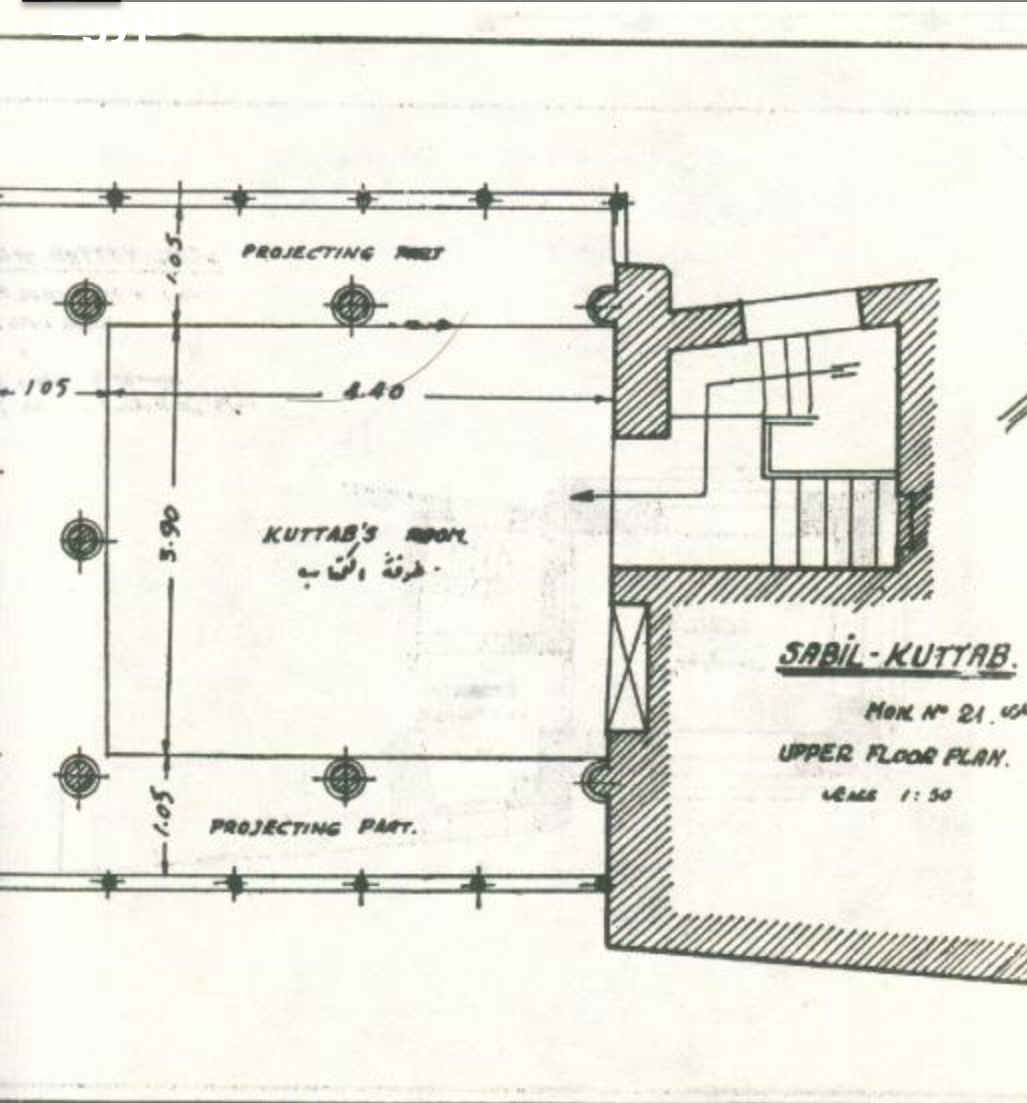
(شكل ١١٥) مسقط الدور الأول لسبيل وكتاب عبد الرحمن كاتخدا بالنحاسين (١٧٤٤م)
